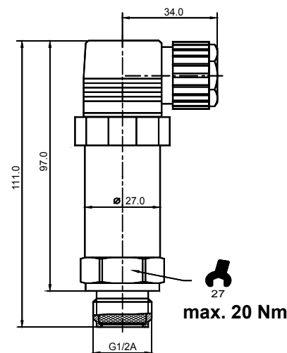
P 20 G 1/2A DIN 3852
