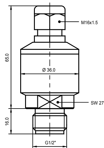
P 115 G1/2A, 11,8 mm Bohrung
